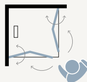
Apertura pieghevole su due lati / 2 folding doors version
