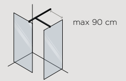
Braccetto a "T" per doppio vetro "T" support arm for double glazing
