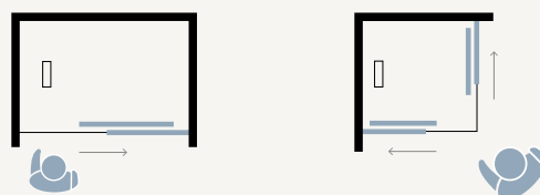
Apertura scorrevole su 2 lati / 2 sliding doors version
