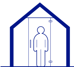
Cerniera vetro su vetro asimmetrico / Glass hinge on asymmetrical glass / Glasscharnier auf asymmetrischem Glas / Charnière en verre sur verre asymétrique
